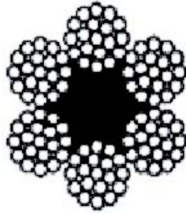
6x19 FC
