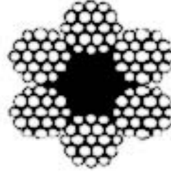
6x19W+FC
