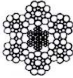
6x19S+IWRC
