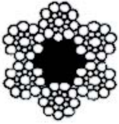
6x19S+FC
