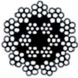
17x7+FC
