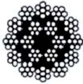
18x7+FC
