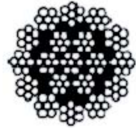
18x7+IWRC
